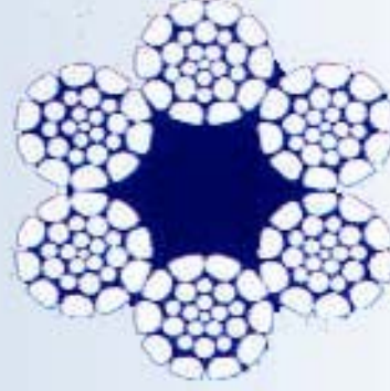
6 x 26WS + IWRC
